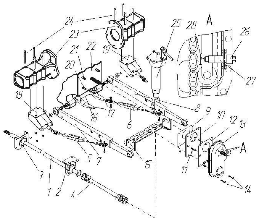
Рисунок 4. Устройство задней навески и ее доработка.
