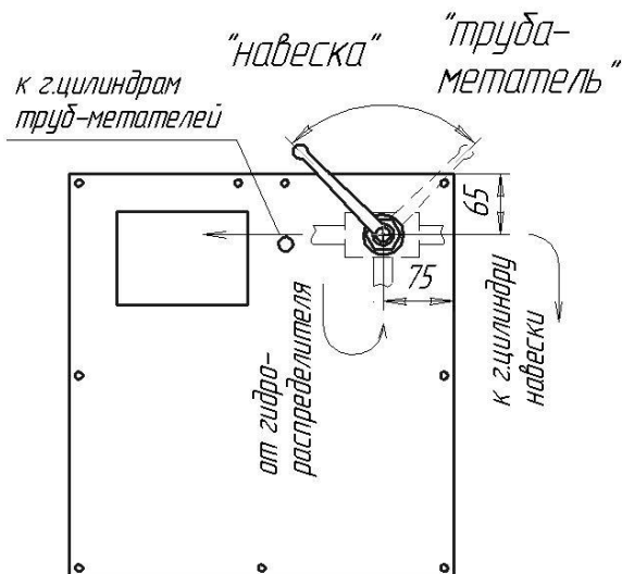
Рисунок 5. Схема расположения трехходового крана.
